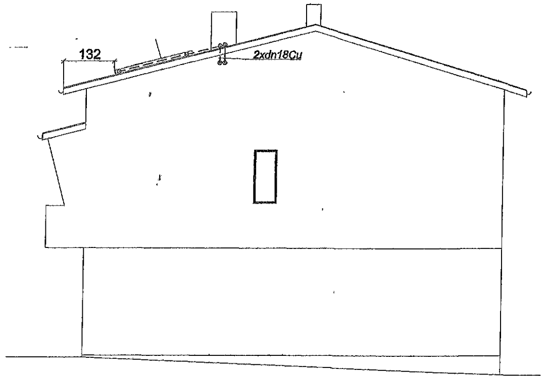
ELEWACJA WSCHODNIA
